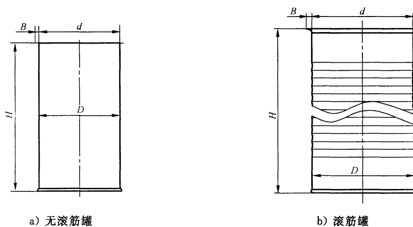
图 2 直身罐
